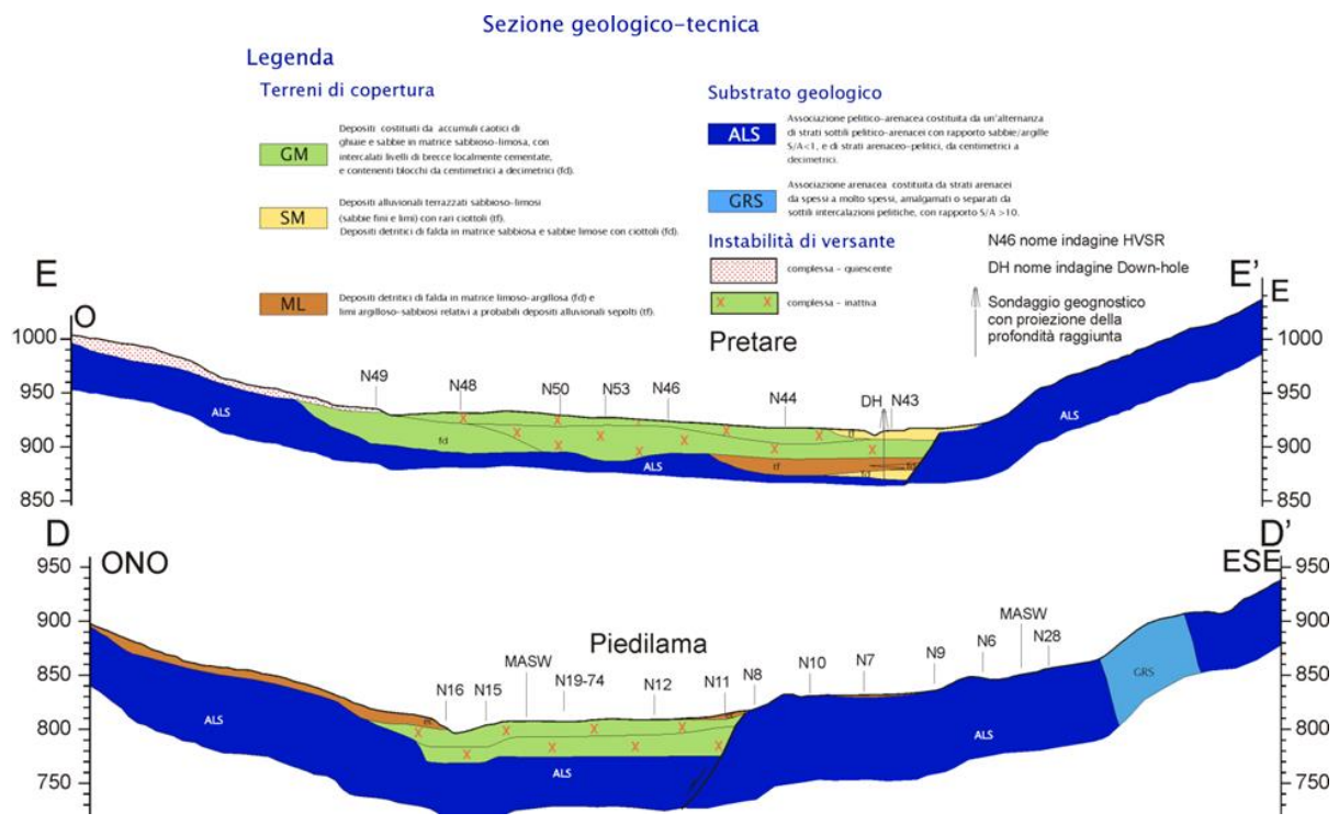
Figura 14 Sezioni Geologico-Tecniche dell'area di Pretare e Piedilama, realizzate nell'ambito degli Studi Microzonazione Sismica di III livello del Comune di Arquata del Tronto.
