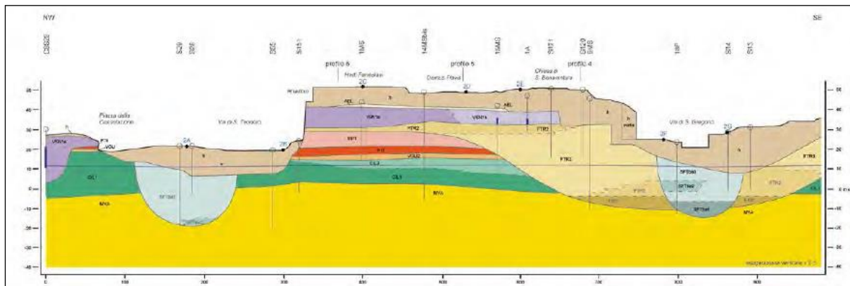
Figura 30 Sezione geologico-technica attraverso l'Area Archeologica Centrale di Roma (M. Palatino). Si noti lo spessore della coltre antropica e l'estensione areale che copre completamente il substrato naturale e le morfologie sepolte (Moscatelli M., 2012)
