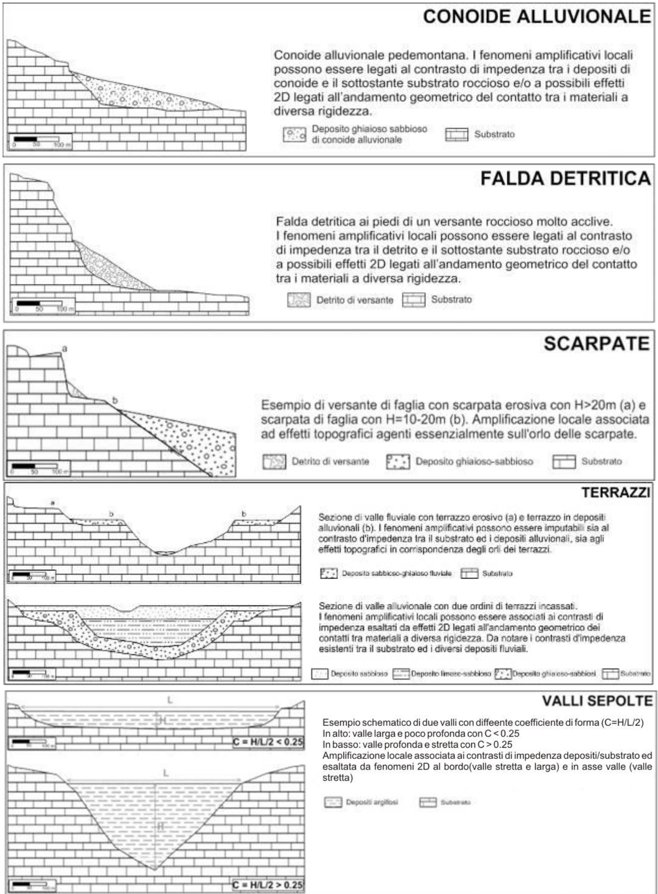
Figura 22 Esempi semplificati di assetti morfologici e geologici che possono condizionare la risposta sismica in superficie.
