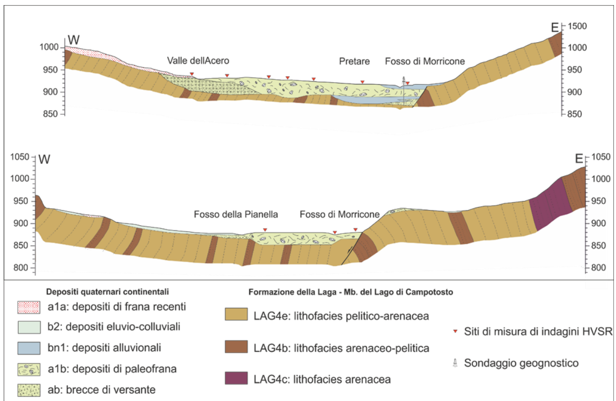
Figura 13 Sezioni geologiche di Pretare in alto e Piedilama in basso realizzate nell'ambito delle attività del Centro per la Microzonazione Sismica e le sue applicazioni, successive all'evento sismico dell'Italia centrale del 24 agosto 2016.
